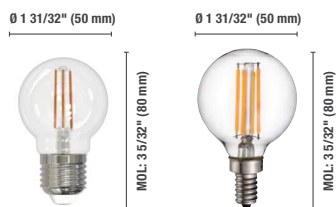
G16.5 5W E26 G16.5 5W E12
